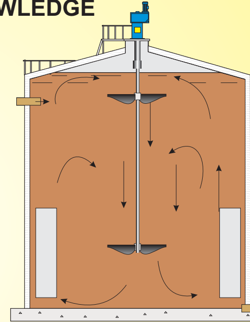
Fermenter
